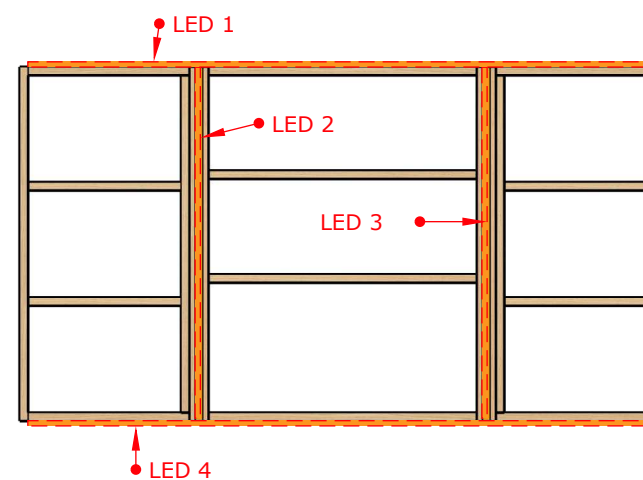
Pohľad spredu - LED pásy
