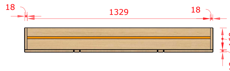
Pohľad spredu - LED pásy
